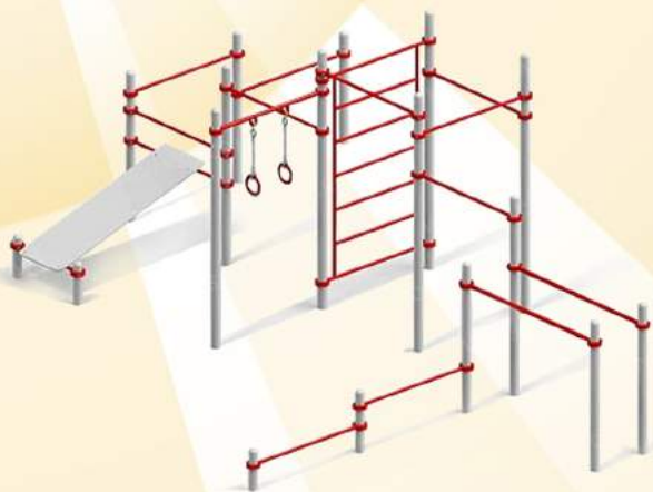
Гимнастический комплекс Workout СП16
